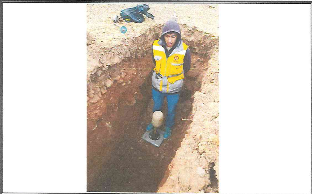
Fotografía N° 12: Vista de la CALICATA N°05; con acercamiento a las paredes de la calicata, señalando la estratigrafía correspondiente. Antes de proceder con el ensayo de densidad en campo.
