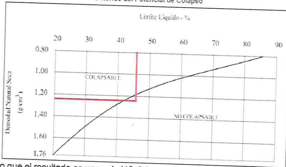
FIGURA 7 Criterios del Potencial de Colapso
