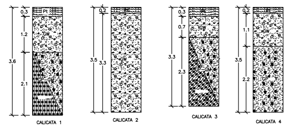
PERFIL ESTRATIGRÁFICO UNIDIMENSIONAL TERRENO 1 ESC: 1/20
