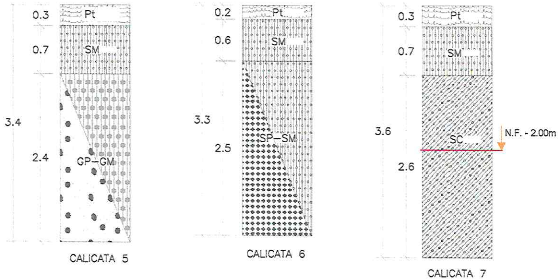
Imagen 11: Perfil Estratigráfico de las calicatas del terreno 2
