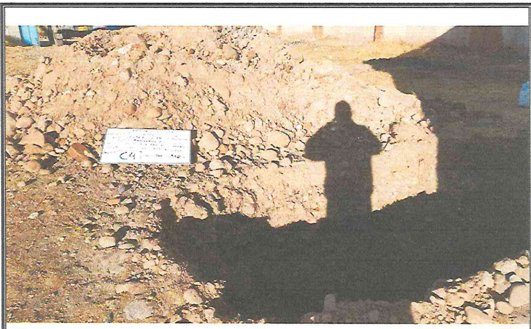
Fotografía N° 08: Vista de la CALICATA N°04 con datos del proyecto; donde se aprecia el material retirado de la exploración; con acercamiento a las paredes de la calicata, señalando parte de la estratigrafía correspondiente.
