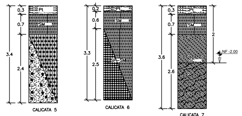
PERFIL ESTRATIGRÁFICO UNIDIMENSIONAL TERRENO 2 ESC: 1/20
