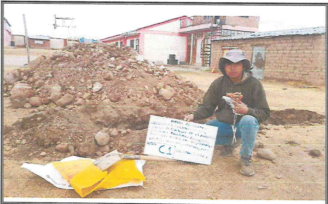
Fotografía N° 02: Vista de la CALICATA N°01 con datos del proyecto; donde se aprecia el material retirado de la exploración.
