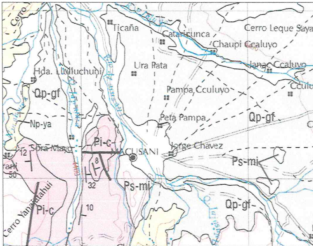
Imagen 06: Mapa Geológico del Cuadrangulo de Macusani 29-v, (Fuente INGEMMET)
