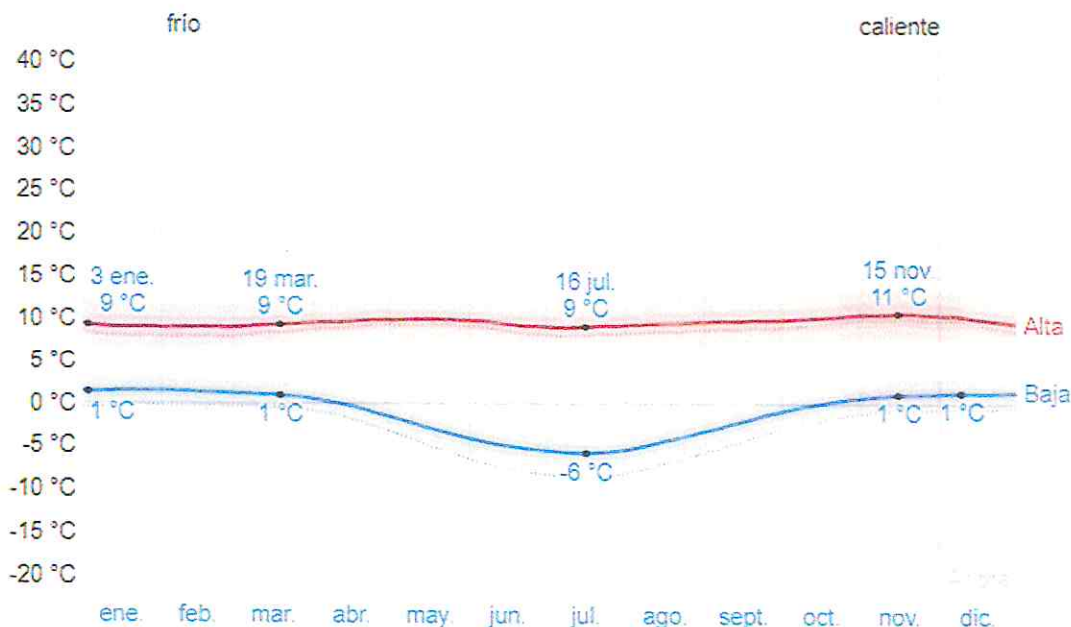
Imagen 05: Temperaturas máximas y mínimas en Macusani
