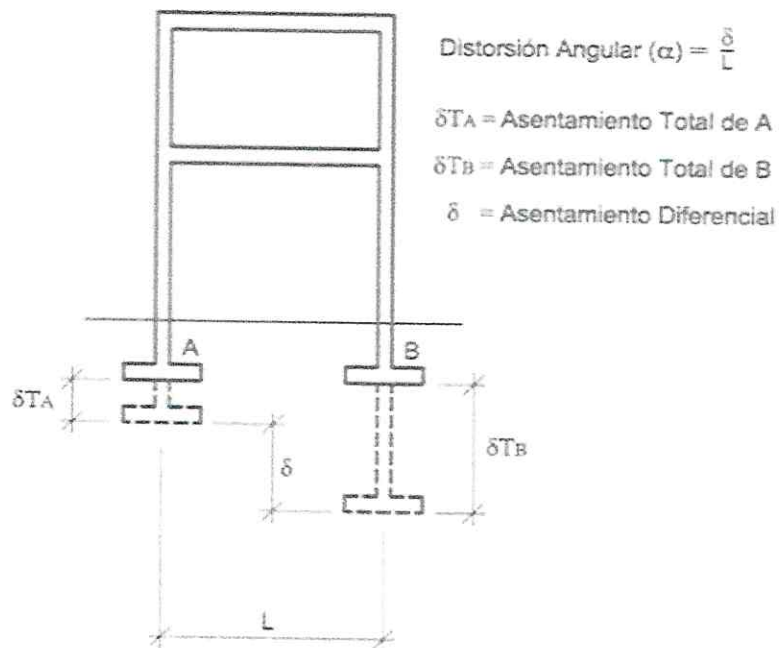
Imagen 13: Distorsión angular
