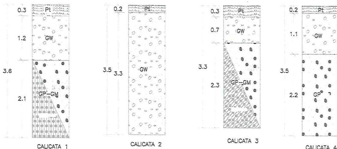
Imagen 10: Perfil Estratigráfico de las calicatas del terreno 1
