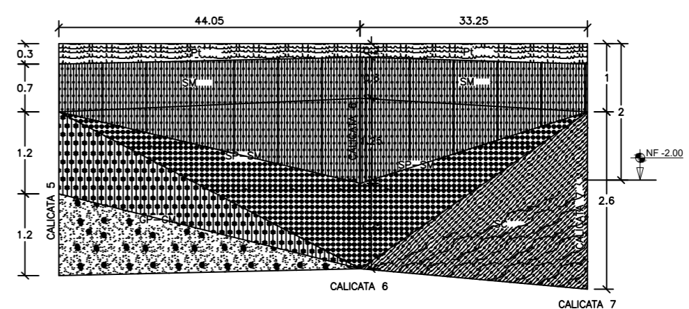
PERFIL ESTRATIGRÁFICO BIDIMENSIONAL TERRENO 2 ESC: 1/20
