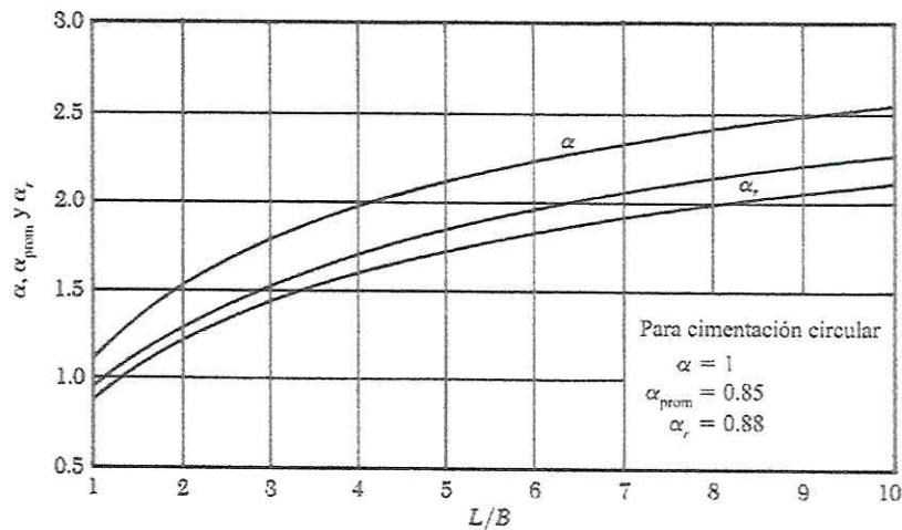
Imagen 12: Parámetros para cálculo de asentamiento
