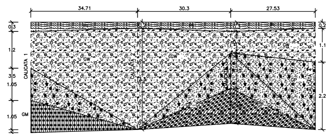
PERFIL ESTRATIGRÁFICO BIDIMENSIONAL TERRENO 1 ESC: 1/20
