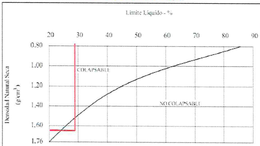
FIGURA 7 Criterios del Potencial de Colapso
