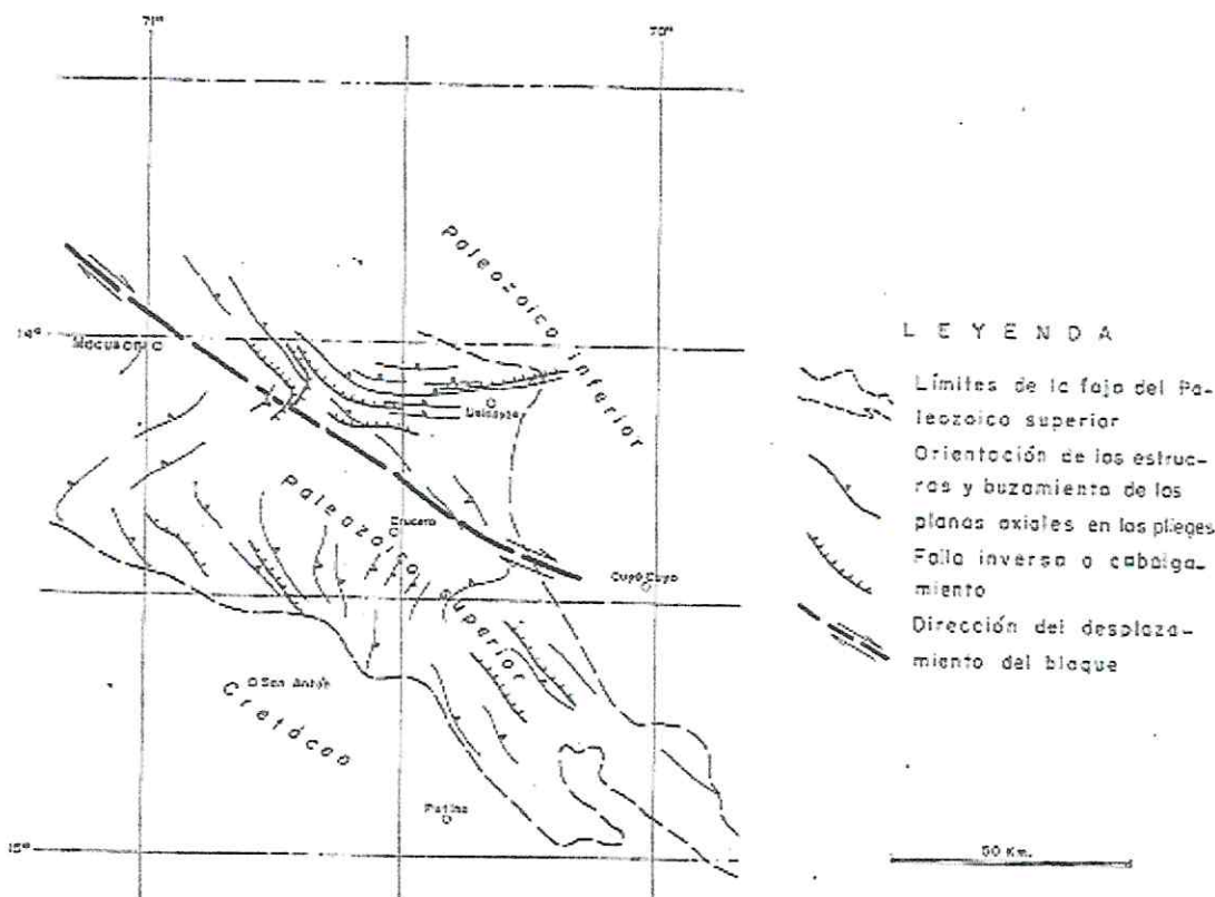
Imagen 09: Leyenda de Mapa Tectónico
