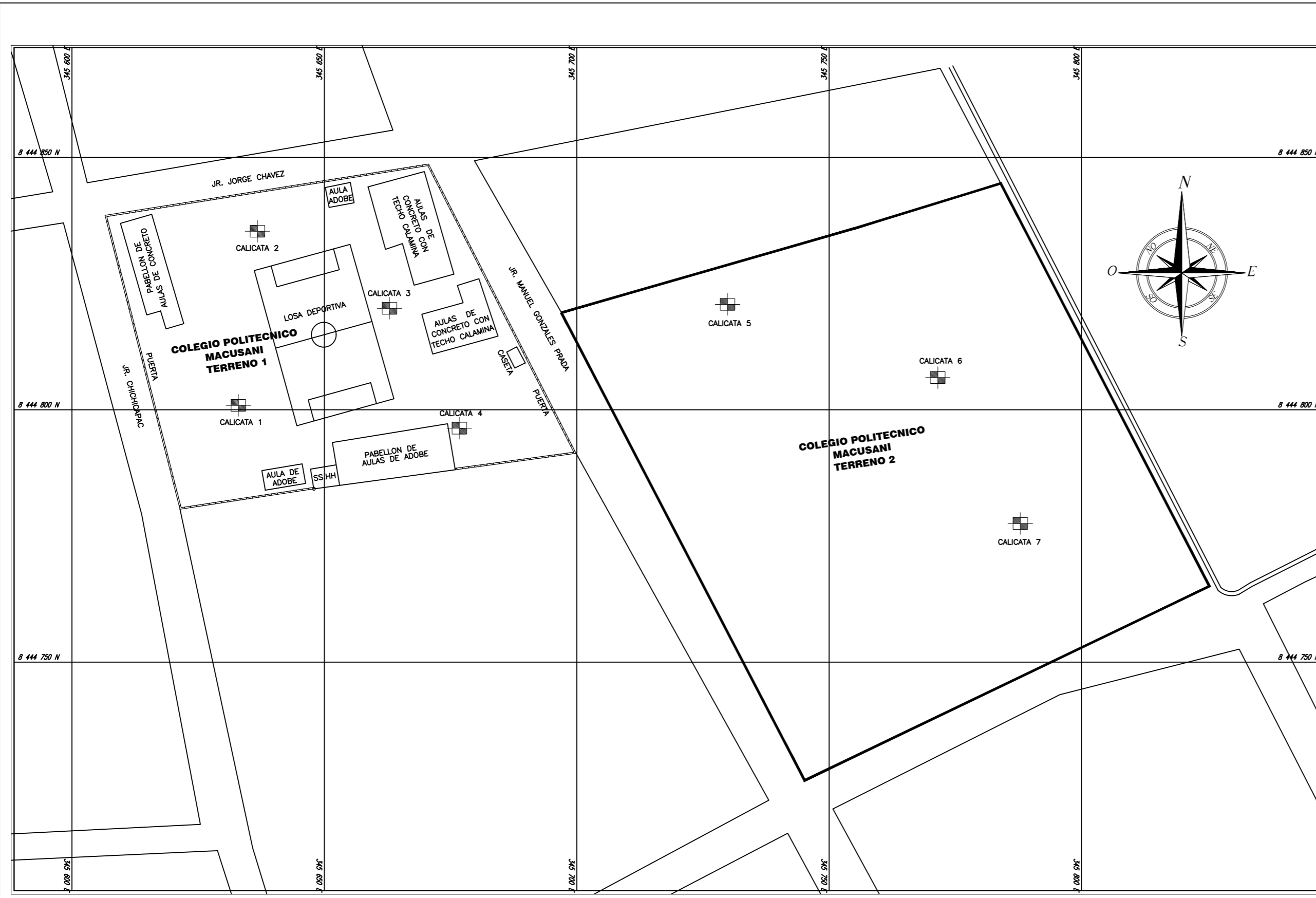
PLANTA DE CALICATAS ESCALA: 1/500
