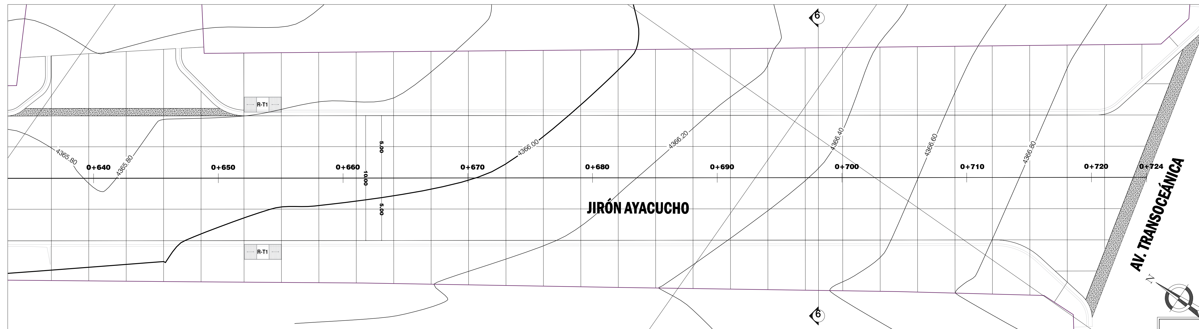
JIRÓN AYACUCHO PROG. 0+640 - 0+724
